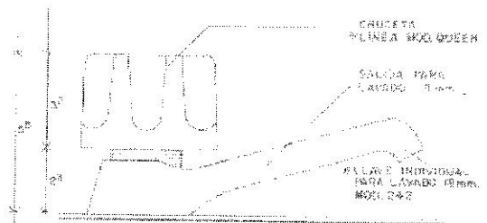
LLAVE INDIVIDUAL PARA LAVABO F MOD 242 (GIGUEN) MISCO URREA E B C 1.1.25
